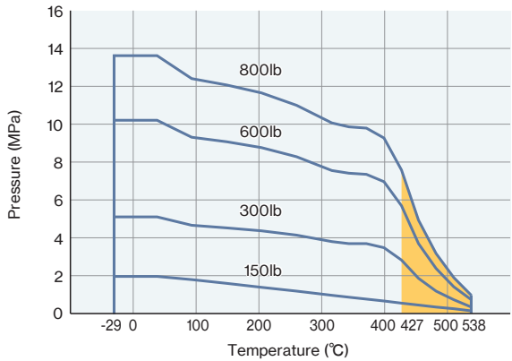
ANSI Valve
