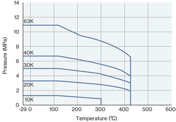
JIS Valve
