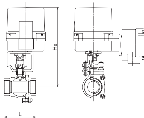
●主要寸法 (単位：mm)
